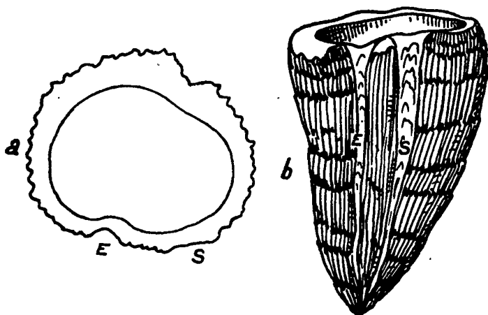
Fig. 1. — Durania delphinensis du Vraconien de la Fauge (échant. n° 1). Valve inférieure; a, vu d'en haut; b, vu latéralement; E, bande siphonale antérieure; S, bande siphonale postérieure. Remarquer l'invagination de la bande E. — Réd. 1/2 environ.
