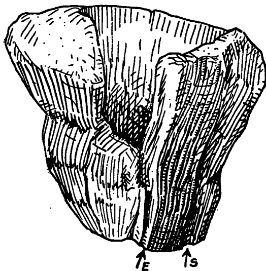
Fig. 2. — Durania delphinensis du Vraconien de la Fauge (échant. n° 2) montrant la grande échancrure du limbe, les bandes excavées E et S et l'interbande saillant. — Réd. 1/2 environ.
